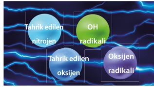
Elektronlar çarpışır ve havadaki nitrojen ve oksijen ile birleşir, neticesinde ise dört tip element ortaya çıkar.
