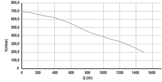
Faydalı Yük - Debi Grafiği
