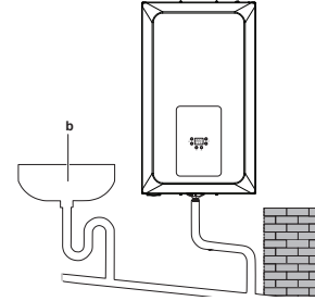
a Ucu açık oluk, yerin altında fakat su seviyesi üstünde
