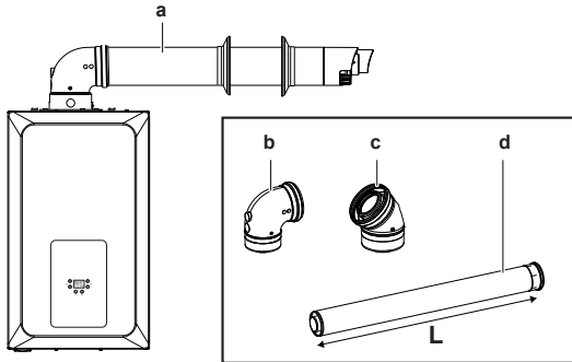
C13x tipi baca
