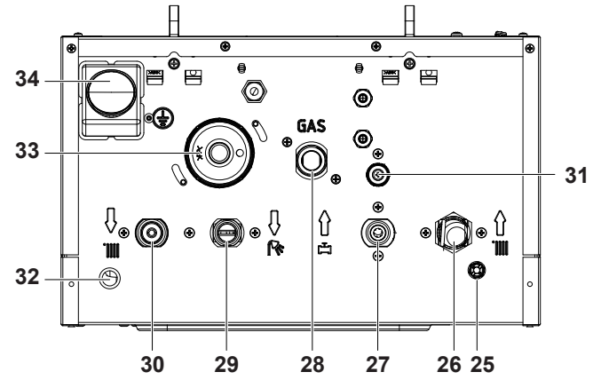
Alt görünüş
