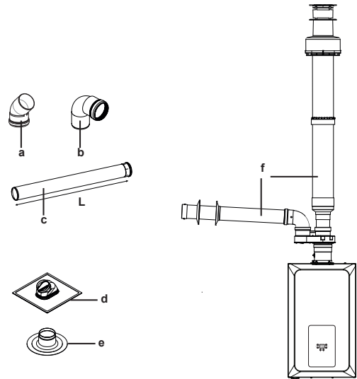
C53x tipi baca
