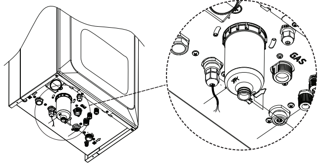
Doldurma vanası ile tesisata su doldurma
